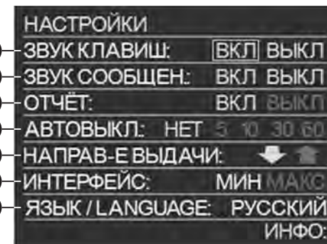
Рис. 4 Заводские установки детектора
